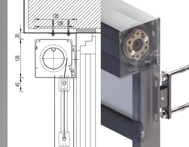
REALSCREEN R95 ZIP - zip sistem sa aluminijumskim vodicama
