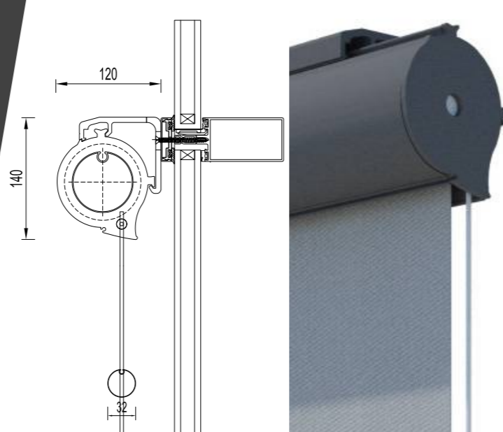
REALSCREEN SK120 - sa zaštitnom kasetom za platno
