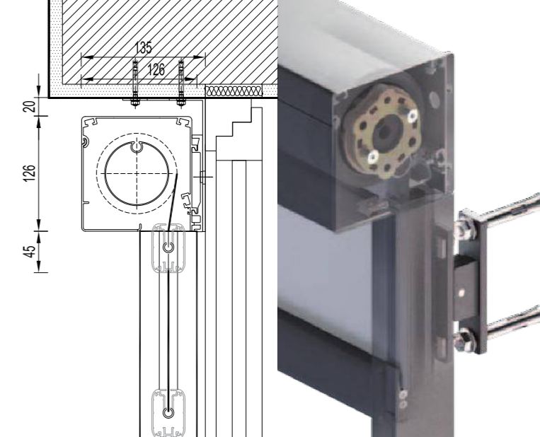
Realscreen R95 ZIP - zip sistem sa aluminijumskim vodicama
