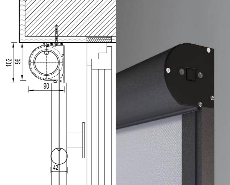
REALSCREEN R76, R90 - za unutrašnju i spoljnu primenu
