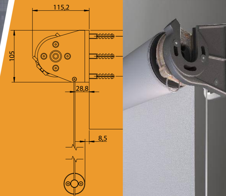
REALSCREEN XL - kabrio screen za unutrašnju i spoljnu primenu
