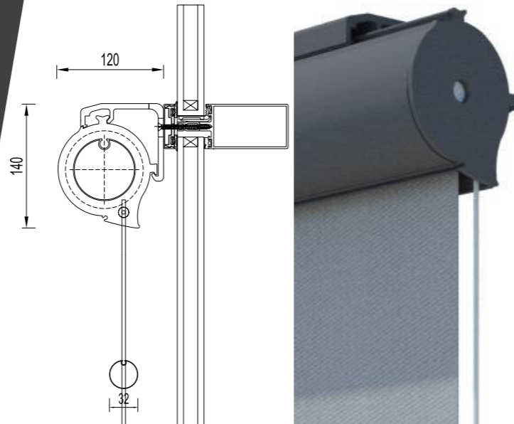
REALSCREEN SK120 - sa zaštitnom kasetom za platno
