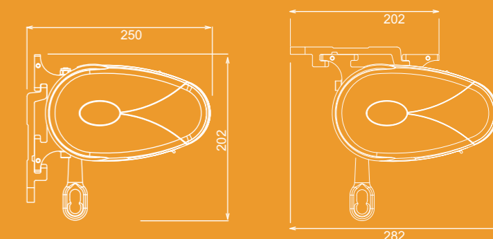
Kasetna tenda - Ugradnja na zid / plafon
