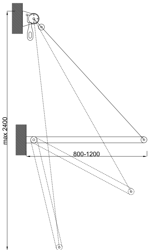
Vertikalna tenda Rodos | Presek
