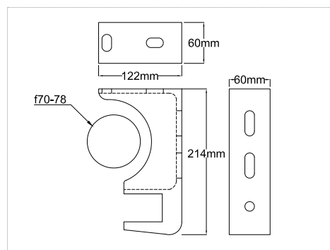
papuča za tendu / awning bracket
